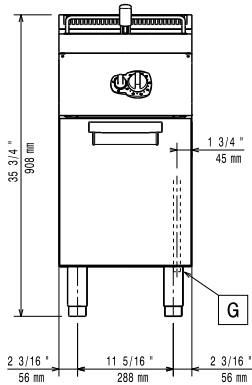
Előlnézet
