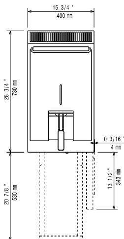
Felülnézet
